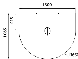
Contura 556, 586, 780 и 880. Угол поворота 90°
