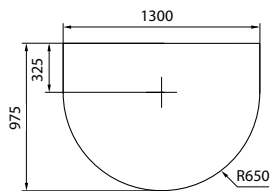
Contura 500 (кроме 556 и 585) и 600. Угол поворота 90°
