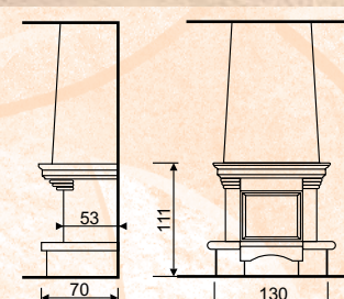
Облицовка FLORA ROSSO с топкой 730 BR
