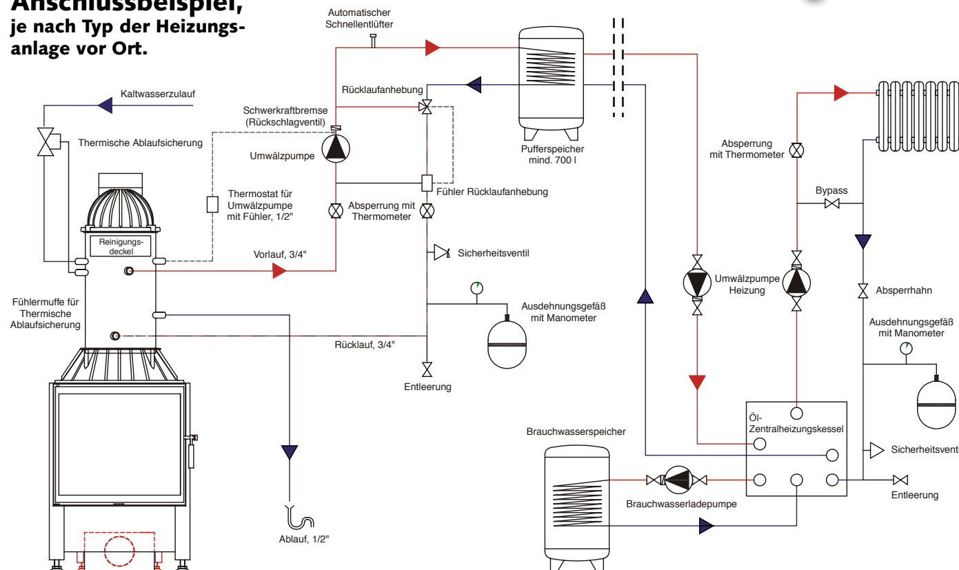
Geschlossener Heizwasser-Kreislauf mit Schmid-Heizwasser-Aufsatzregister für Kamineinsätze und Öl-/Gaskessel (Zentralheizung)
