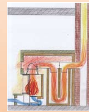
Schmid-Feuerungstechnik als Kaminanlage mit keramischer Nachheizfläche.
