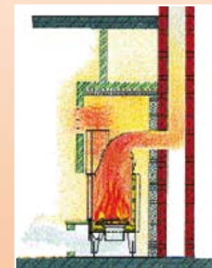
Schmid-Feuerungstechnik als Wamluft-Kaminanlage.
