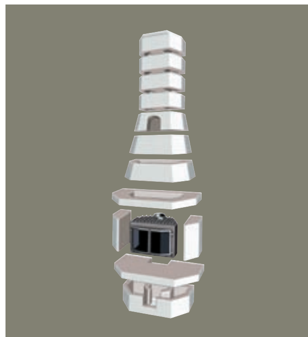
Каменные печи Keddy поставляются в виде легко собираемых комплектов, состоящих из отдельных секций из пемзы.
