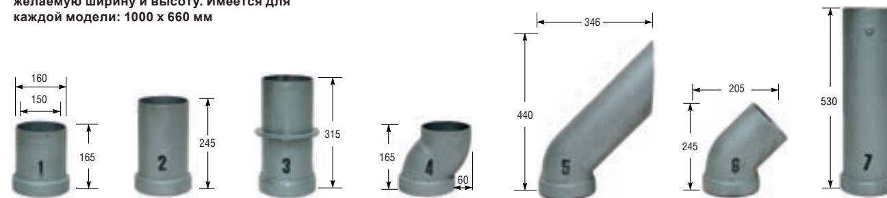
Чугунные трубы для каминных вставок Keddy для подсоединения к существующему дымоходу. Размеры в мм.
